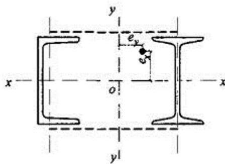
Рисунок 5 - Схема стержня сквозного сечения из двух сплошнотенчатых ветвей
