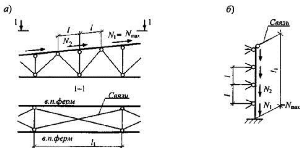
а - пояс фермы; б - ветвь колонны
