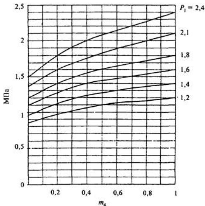
График для определения давления в изотермическом резервуаре в конце выпуска расчетного количества двуокси углерода
