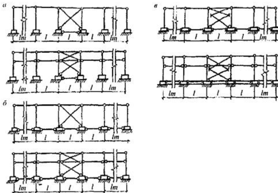
а - е - типы соединений элементов каркаса
