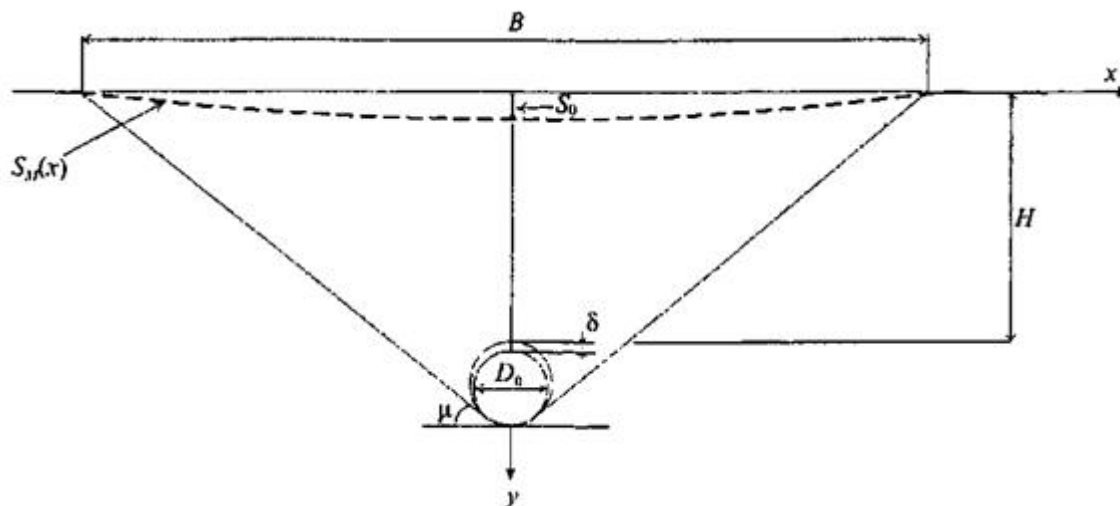
Рисунок А.1 - Иллюстрация видов сдвижений и деформаций земной поверхности при разработке пластового месторождения
