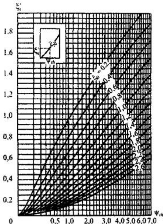
Рисунок K.5 - Графики для определения коэффициента \xi'_c
