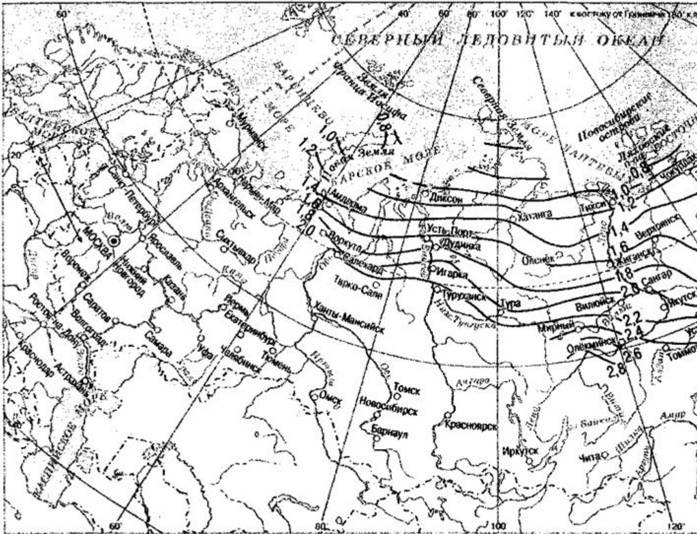
Рисунок Г.2 - Глубины оттаивания глинистых грунтов
