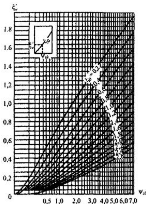
Рисунок К.6 - Графики для определения коэффициента \xi'_{\epsilon}
