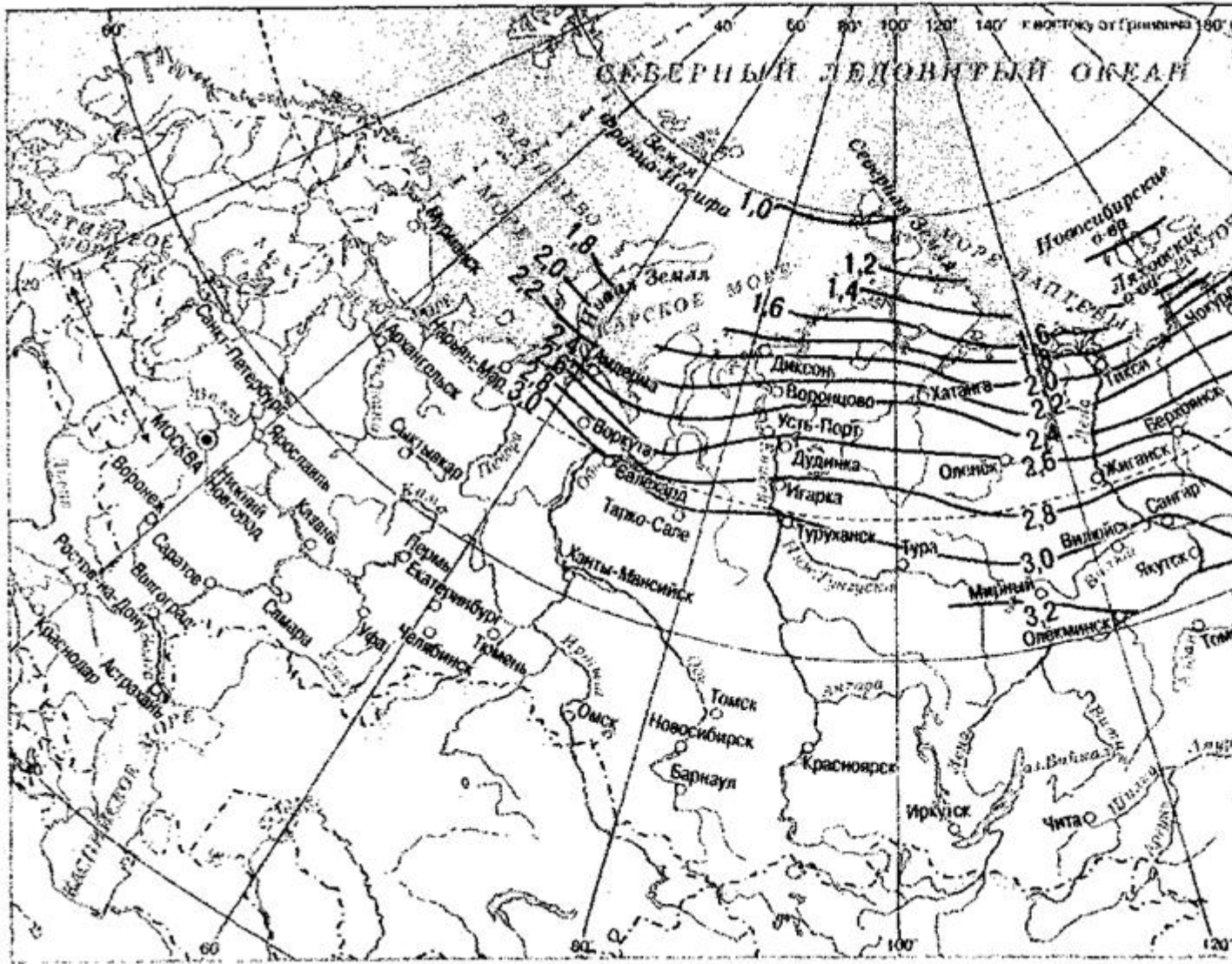
Рисунок Г.1 - Глубины оттаивания песчаных грунтов
