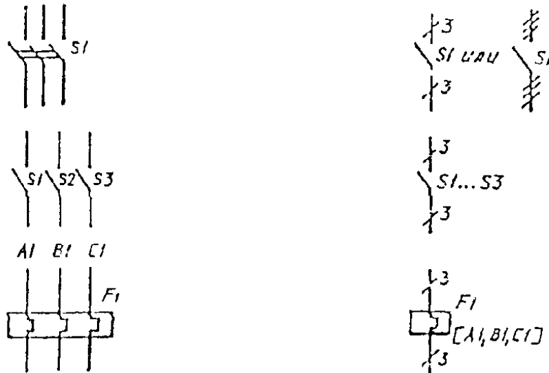
а - многолинейное изображение; б - однолинейное изображение.
