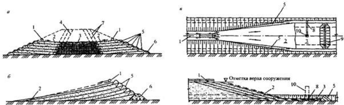
Рисунок 4 - Виды намывных плотин
