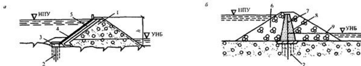
Рисунок 8 - Виды взрывонабросных плотин
