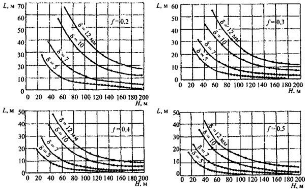
Рисунок Ж.1 - Зависимость расстояния между горизонтальными швами диафрагмы по высоте L , от толщины диафрагмы \delta , величины коэффициента трения грунта по диафрагме f и высоты диафрагмы H
