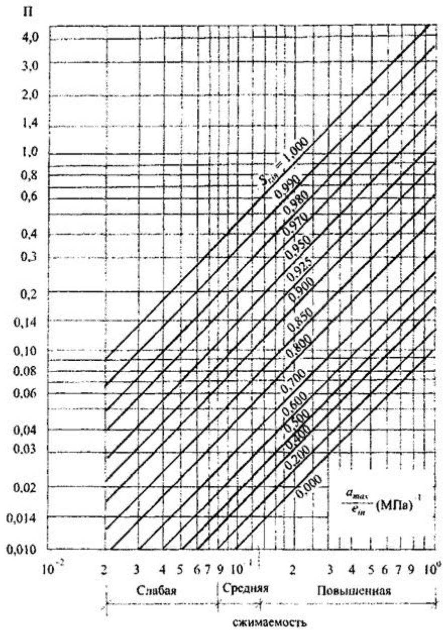
Рисунок А.2 - Номограмма для определения параметра П
