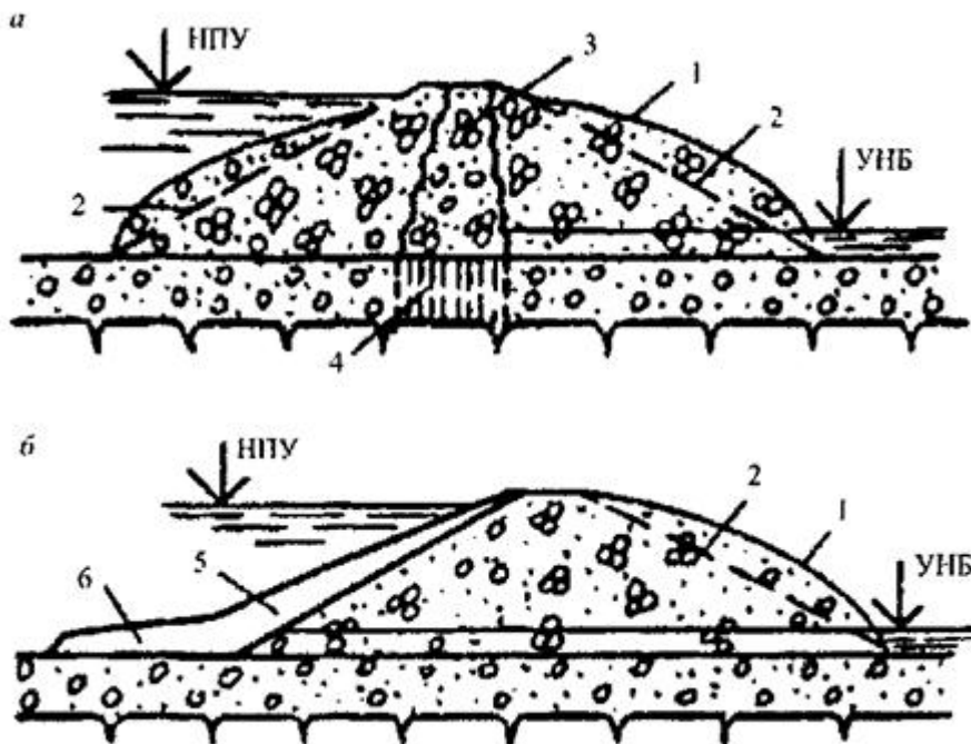
Рисунок 7- Виды каменно-земляных плотин
