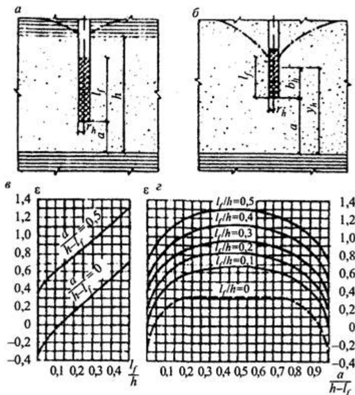
а, б - схемы несовершенных скважин в напорном и безнапорном пластах; в, г - графики для определения \epsilon
