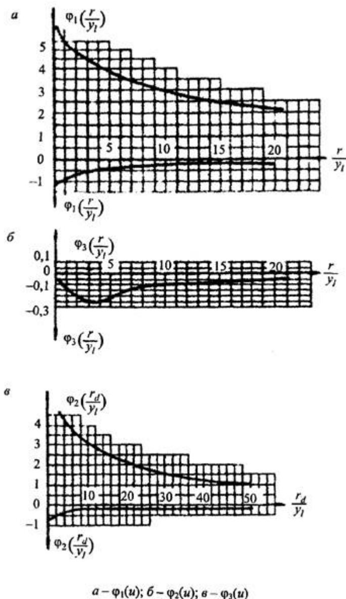
Рисунок А.5 - Графики функций
