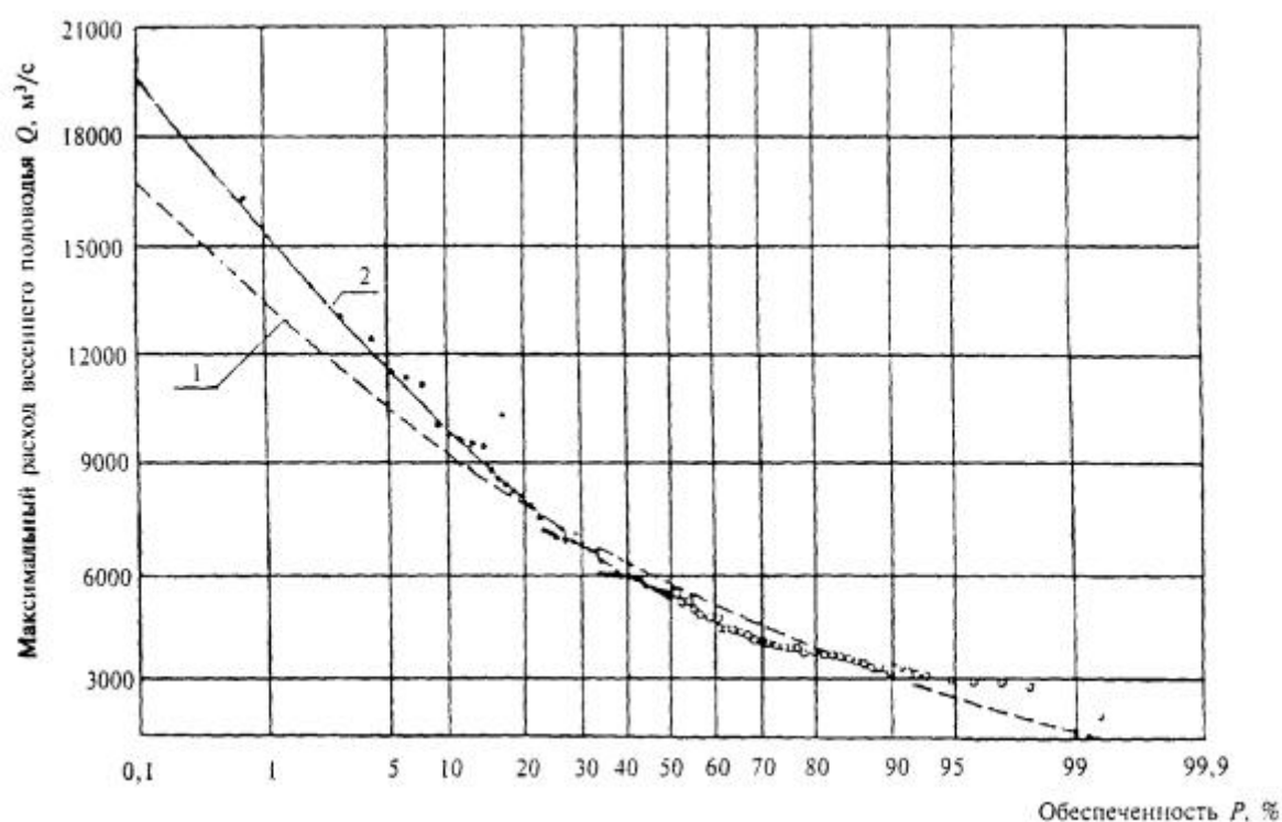
Гамма-распределение: 1 - полное; 2 - усеченное
