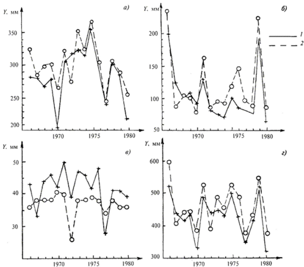
Рисунок А.5 - Сравнение фактических (1) и рассчитанных (2) слоев стока р. Вага - с. Усть-Сюма
