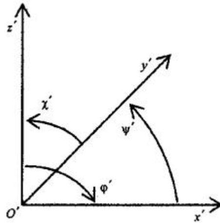
Рисунок Б.1 - Степени свободы фундамента
